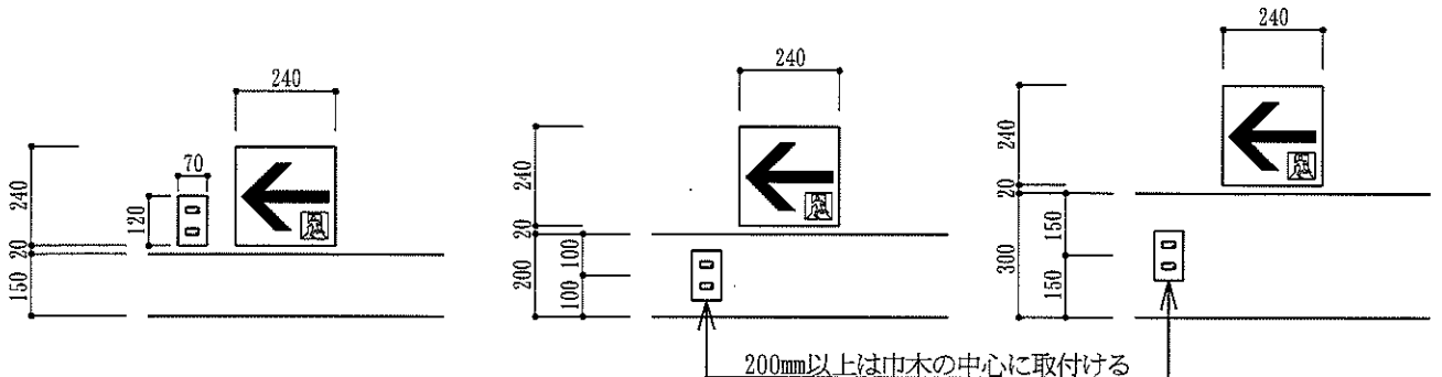
廊下におけるコンセント及び誘道灯取付け高さ位置
